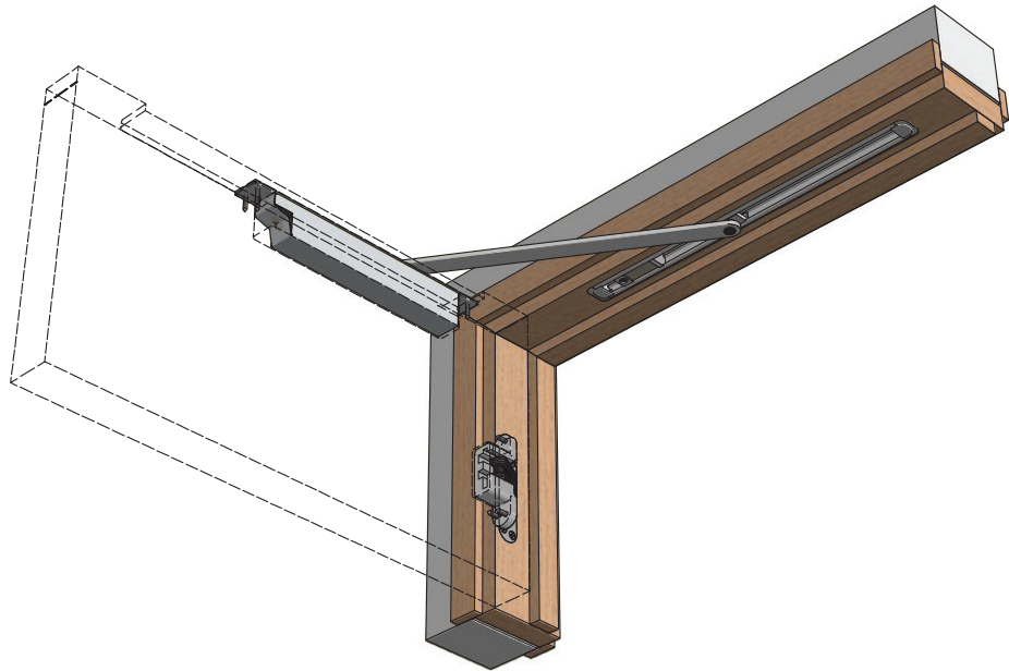
Perspective - door open
