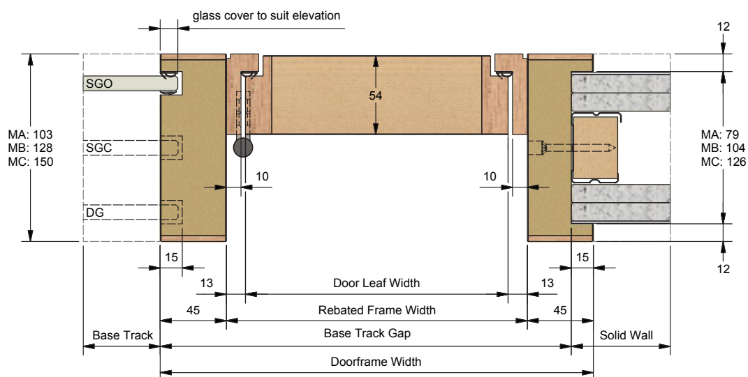
Door Jambs (1:3)
