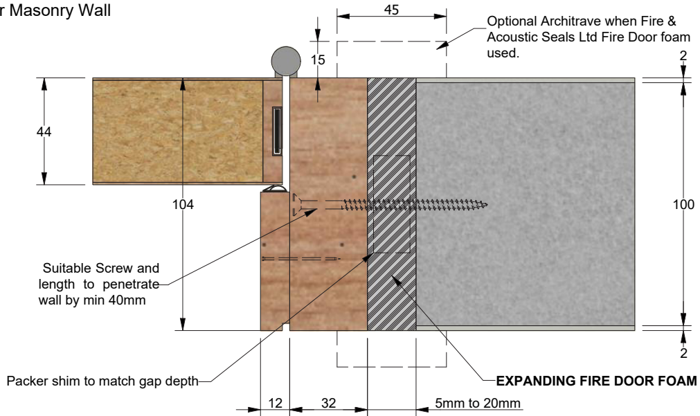
FD30 Door Masonry Wall
