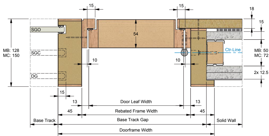
Door Jambs (1:3)
