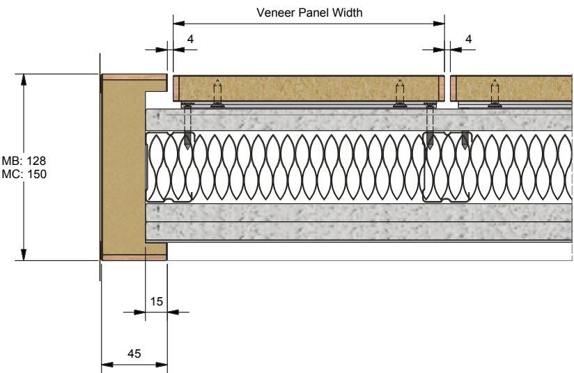
Door Jambs (1:3)
